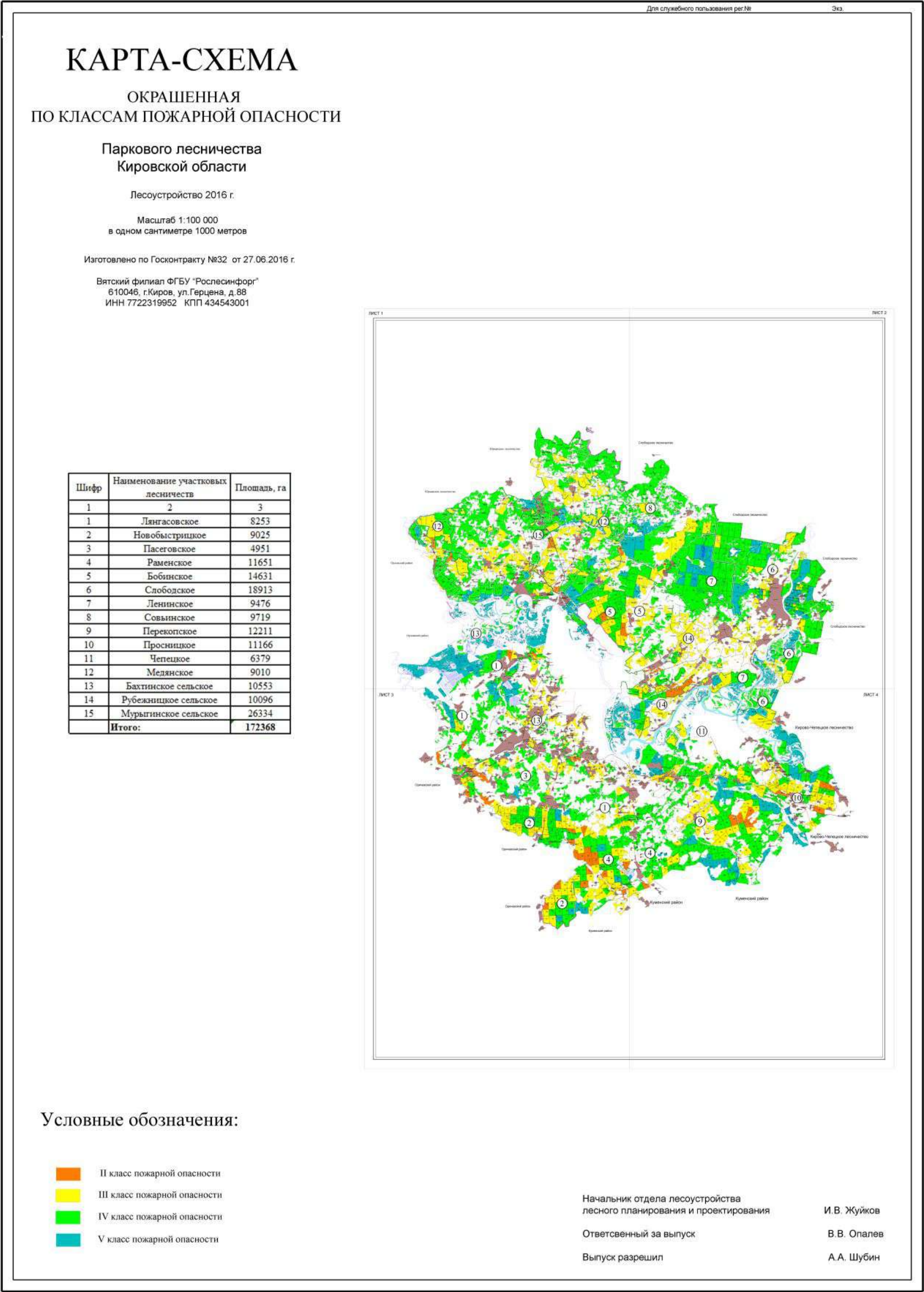
Рисунок 5 Карта схема классов пожарной опасности Паркового лесничества
