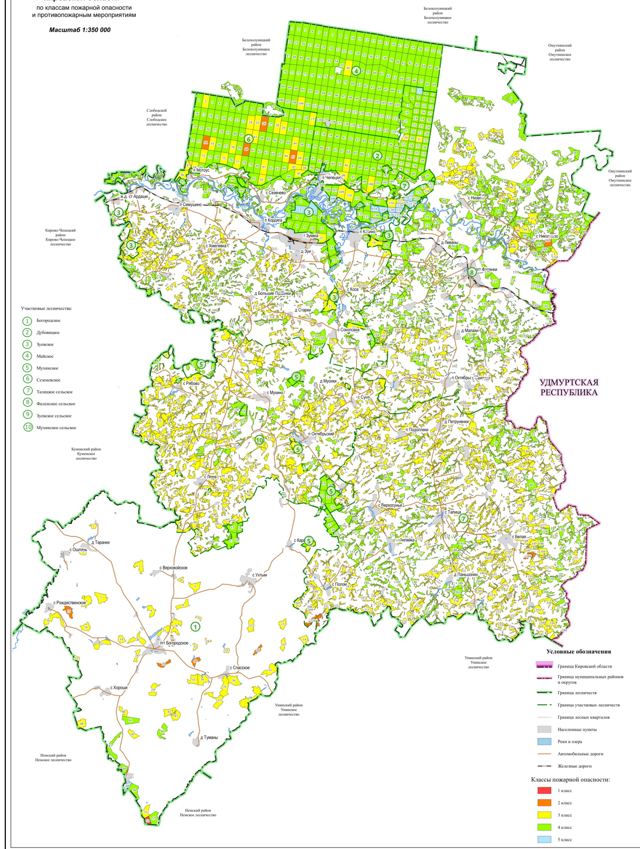
Рисунок 5. Карта-схема распределения площади лесов по классам пожарной опасности Зуевского лесничества
